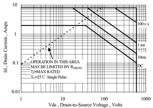
图 6 最大安全工作区曲线
